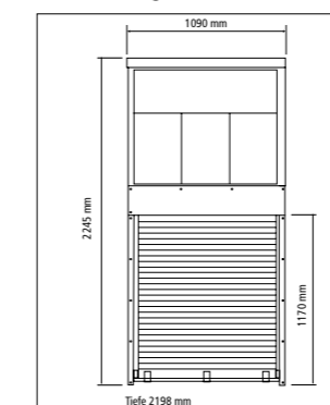
Erweiterungsmodul 3
