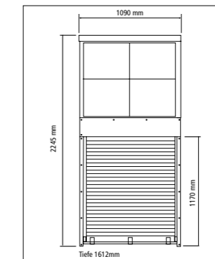
Erweiterungsmodul 4
