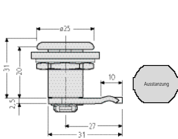
Zylinderschloss ER 97-9-95276 17,00 € Schließung 1-50 inkl. 2 Schlüssel, für Modellgruppe 60, 62 und 63 (RENZ PLAN) Einbau ab 2010, mit Mutter und Dichtung
