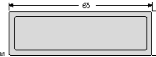
Namensschild 97-9-82178 16,70 € Größe 65 x 20 mm, Ausstanzung 60,8 x 17,8 mm Verkauf solange Vorrat reicht.
