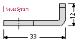
Riegel gekröpft – Auslaufmodell – für 3-Punkt-Verriegelung Serienkästen 97-9-95014 5,40 €
