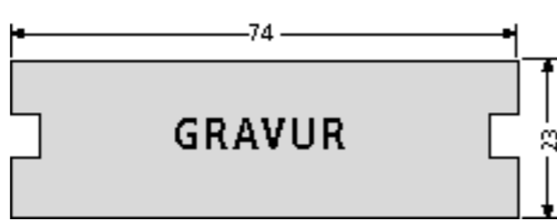
Namensschildleinlage Kunststoff für 97-9-00211 und 97-9-00212, Hintergrundfarbe schwarz oder weiß
