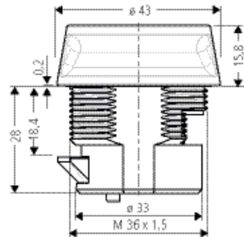
Zylinderschloss 225-024 , Schließung 2C 100 *97-9-95061 inkl. 2 Schlüssel, Einbau für Mitteilungskasten Modellgruppe 30, ohne Riegel
