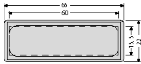
Namensschild – Einbau ab 1978 – 97-9-82033 5,00 € für Klappe nach außen aufgehend. Namensschildleinlage max. 60 x 15 x 0,5 mm, Ausstanzung 61 x 18 mm
