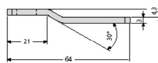
Riegel für Paketkasten , für „Schwere Baureihe“ 97-9-00437 5,40 €
