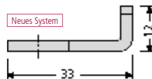
Riegel gekröpft – Auslaufmodell – für verstärkte Tür 97-9-95011 2,90 €
