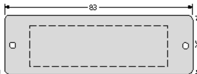
ALU-Namensschildplatte EV1 – Einbau ab 1987 – 97-9-00211 17,30 € innen, Antivandalismus, Namensschildleinlage max. 74 x 23 x 0,5 mm, Ausstanzung 61 x 18 mm
