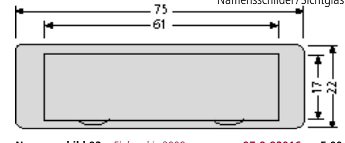
Namensschild 92 – Einbau bis 2009 – 97-9-82016 5,00 € 75 x 22 mm glasklar/0000 oder mit grauem Rand/7039 (bei Bestellung bitte angeben), Namensschildleinlage max. 60 x 15 x 0,5 mm, Ausstanzung 71 x 19 mm glasklar/0000 oder grau/7039
