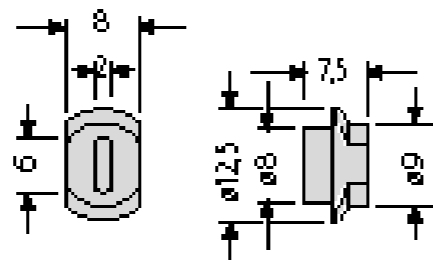
Namensschildsperrle – Einbau ab 1982 – 97-9-82035 2,30 € passend zu 97-9-82033
