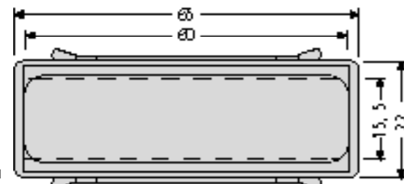
Namensschild 97-9-00302 5,00 € mit Feder für Einbau in Türen, Namensschildleinlage max. 60 x 15 x 0,5 mm, Ausstanzung 61 x 18 mm
