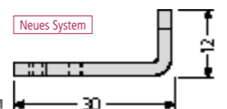
Riegel gekröpft für neues System mit Befestigungsfeder (Standard-Briefkästen) 97-9-00363 2,90 €
