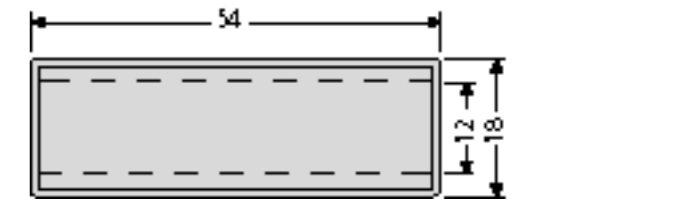
Namensschild – Einbau ab 1970 – 97-9-82014 5,00 € für Durchwurfschal, Namensschildleinlage max. 50 x 12 x 0,5 mm, Ausstanzung 50 x 14 mm
