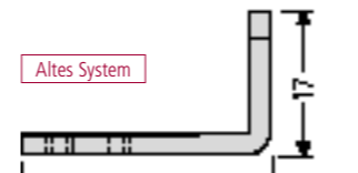
Riegel gekröpft für altes System mit Befestigungsfeder (Standard-Briefkästen) 97-9-00364 2,90 €
