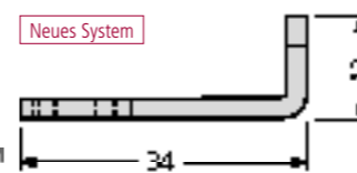
Riegel gekröpft für verstärkte Tür oder 2/3-Punkt-Verriegelung mit Befestigungsfeder 97-9-00361 5,40 €
