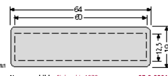
Namensschild – Einbau bis 1978 – 97-9-82019 5,00 € 64 x 19 mm, für 2,5 mm Materialdicke, zum Einklippen, Namensschildleinlage max. 59,5 x 12,5 x 0,5 mm, Ausstanzung 60 x 15 mm
