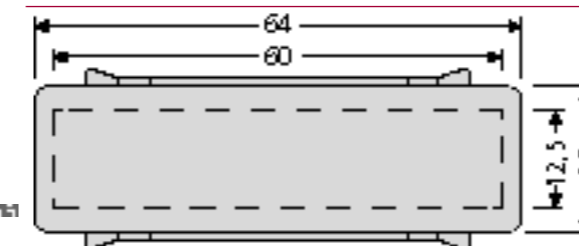
Namensschild 97-9-00303 5,00 € 64 x 19 mm, mit Feder Namensschildleinlage max. 60 x 12,5 x 0,5 mm, Ausstanzung 60 x 15 mm. Einbau für altes Modell: 11-409, 11-410, 12-451, 15-000, 17-200, 17-419, 17-425
