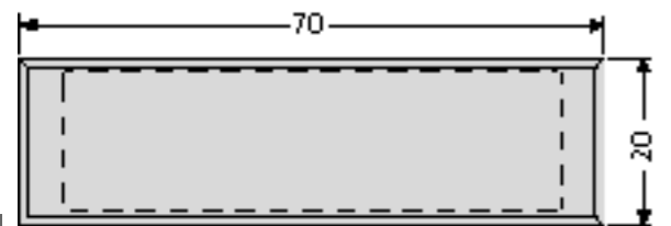
Namensschild 97-9-82173 6,40 € 70 x 20 mm, Ausstanzung 67 x 17 mm. Verkauf solange Vorrat reicht.
