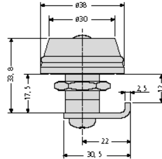
Kombinations-Zahlenschloss 97-9-95238 54,90 € aus Metall, Farbe schwarz nach Eingabe des 3-stelligen Codes lässt sich das Schloss entriegeln.
